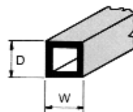
Tubes en ABS gris clair ST- de section carrée
