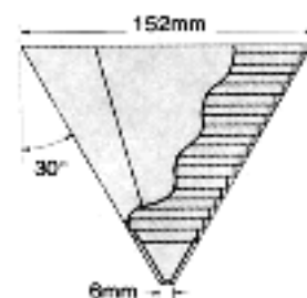
Cône à 60° en ABS gris - diamètre = 152,00mm
