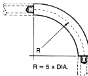
Coude (5xD) à 90° en butyrate de couleur -() - pour tubes P-()
