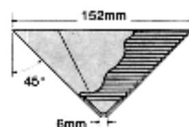
Cônes à 45° en ABS gris moulé - diamètre = 152,00mm
