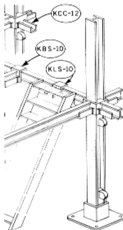
Exemple d'assemblage de poutres en H sur embase
