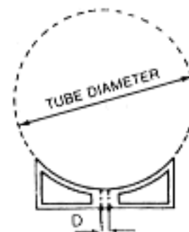
Berceau en ABS gris pour tubes de couleur P()- ou VT-
