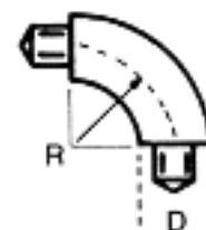
Calcul du rayon par rapport au diamètre des tubes P()-
