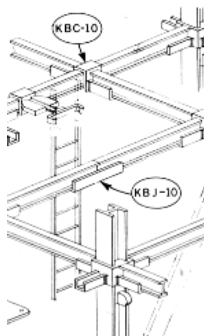
Exemple d'assemblages de poutres en H et en I par emboîtement
